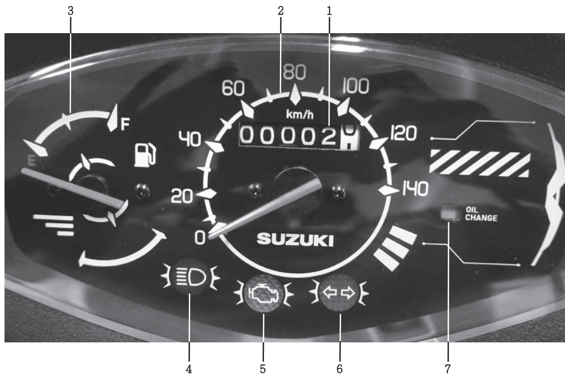
1.里程表 2.速度表 3.油量表 4.遠光指示燈 5.引擎故障燈 6.方向指示燈 7.機油更換指示器
